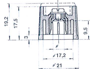
mit Strich — avec repère — with line
